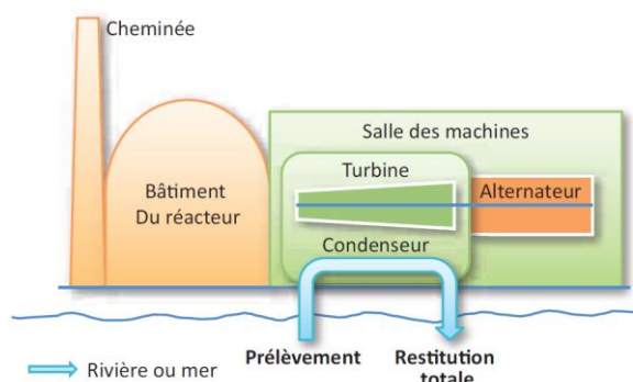
Figure 3 : Schéma d'un CNPE avec un circuit de refroidissement ouvert (Source : EDF)
