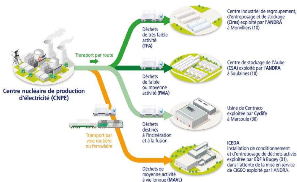
Figure 4 : Transport des déchets radioactifs (Source : EDF)
