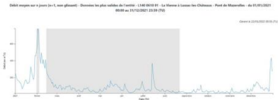
Figure 4-2. Hydrologie de la Vienne à la station de Lussac-les-Châteaux pour l'année 2021 (Qjm : débit moyen journalier en \text{m}^3.\text{s}^{-1} ; QMM : débit moyen mensuel en \text{m}^3.\text{s}^{-1} )
