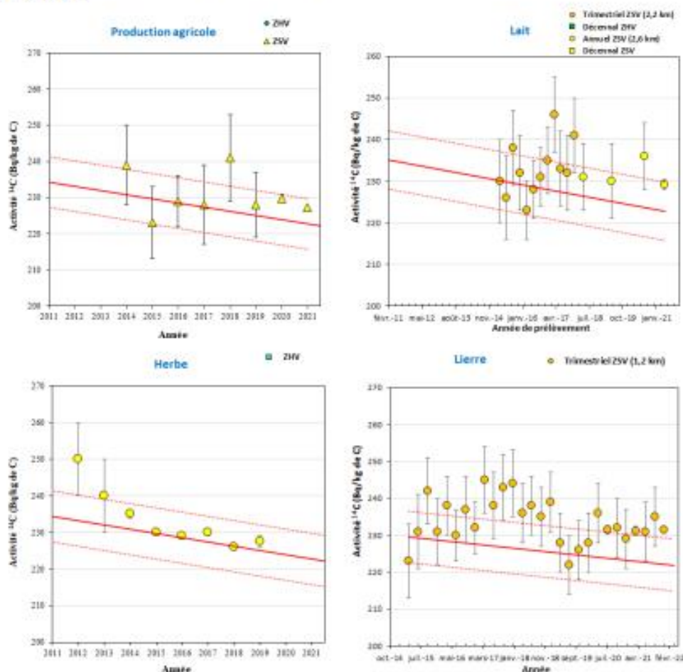
Figure 5-6. Activités spécifiques en ^{14}\text{C} mesurées dans les échantillons prélevés dans l'environnement terrestre du C.N.P.E. de Belleville-sur-Loire de 2011 à 2021.
