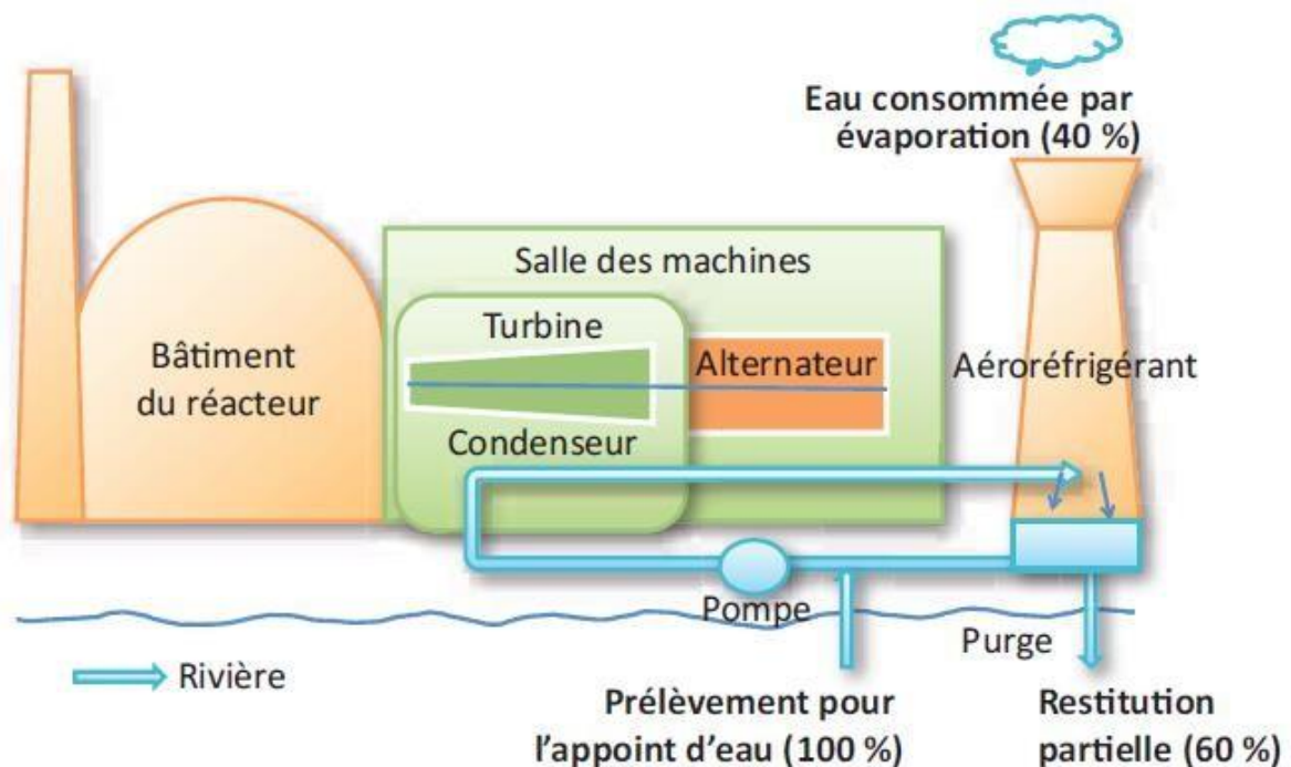
Figure 3 : Schéma d'un CNPE avec un circuit de refroidissement fermé (Source : EDF)
