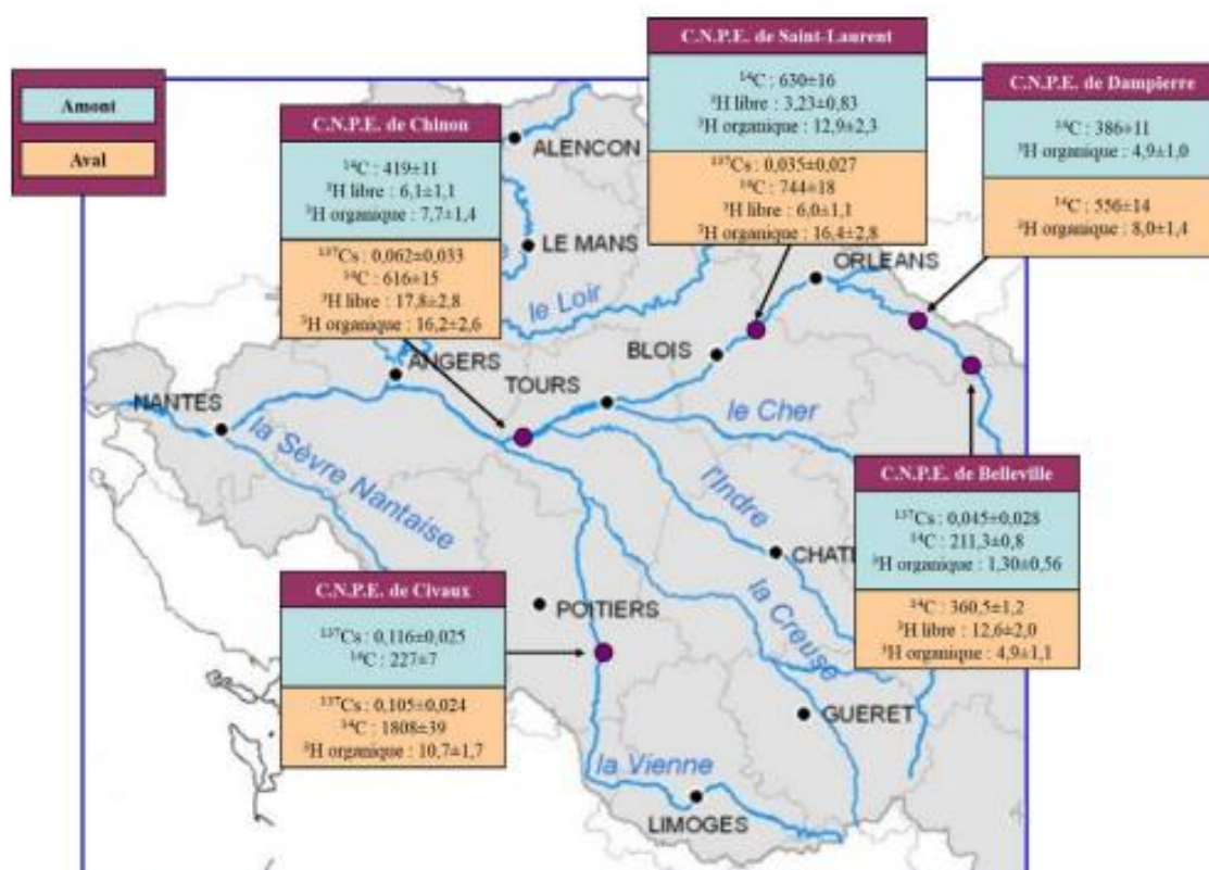
Figure 10-5. Synthèse des activités des radionucléides artificiels, du ^{14}\text{C} et du ^3\text{H} détectés dans les poissons prélevés en 2021 dans l'environnement des C.N.P.E. du bassin de la Loire.
