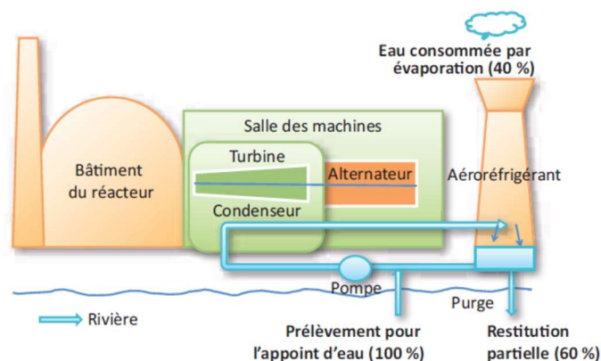
Figure 1 : Schéma d'un CNPE avec un circuit de refroidissement fermé
