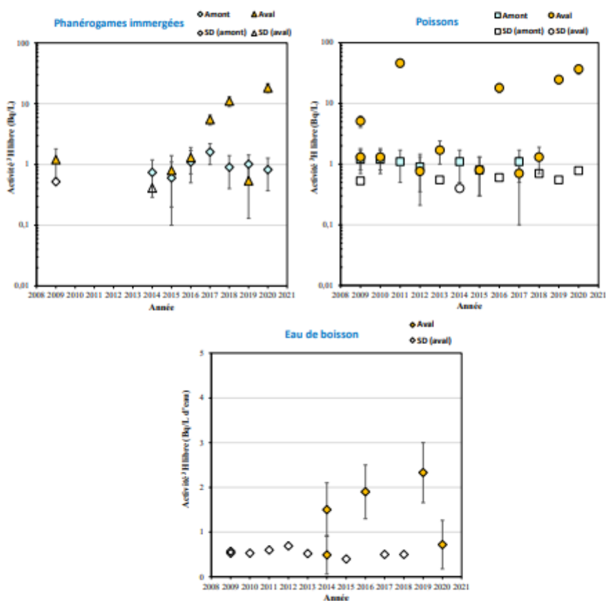
Figure 5-11. Activités en tritium libre dans les échantillons prélevés dans l'environnement aquatique du C.N.P.E. de Belleville-sur-Loire de 2009 à 2020.
