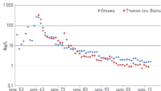
Figure 3-1. Evolution temporelle de l'activité en tritium de l'eau de pluie dans l'hémisphère Nord (Ottawa et Thonon-les-Bains) depuis 1955 [27].
