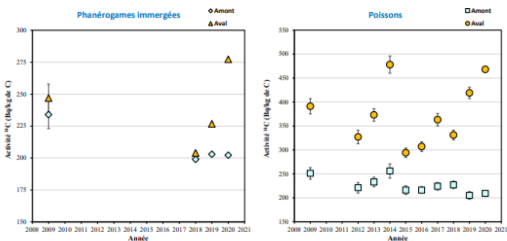
Figure 5-13. Activités spécifiques en ^{14}\text{C} dans les échantillons prélevés dans l'environnement aquatique du C.N.P.E. de Belleville-sur-Loire de 2009 à 2020.
