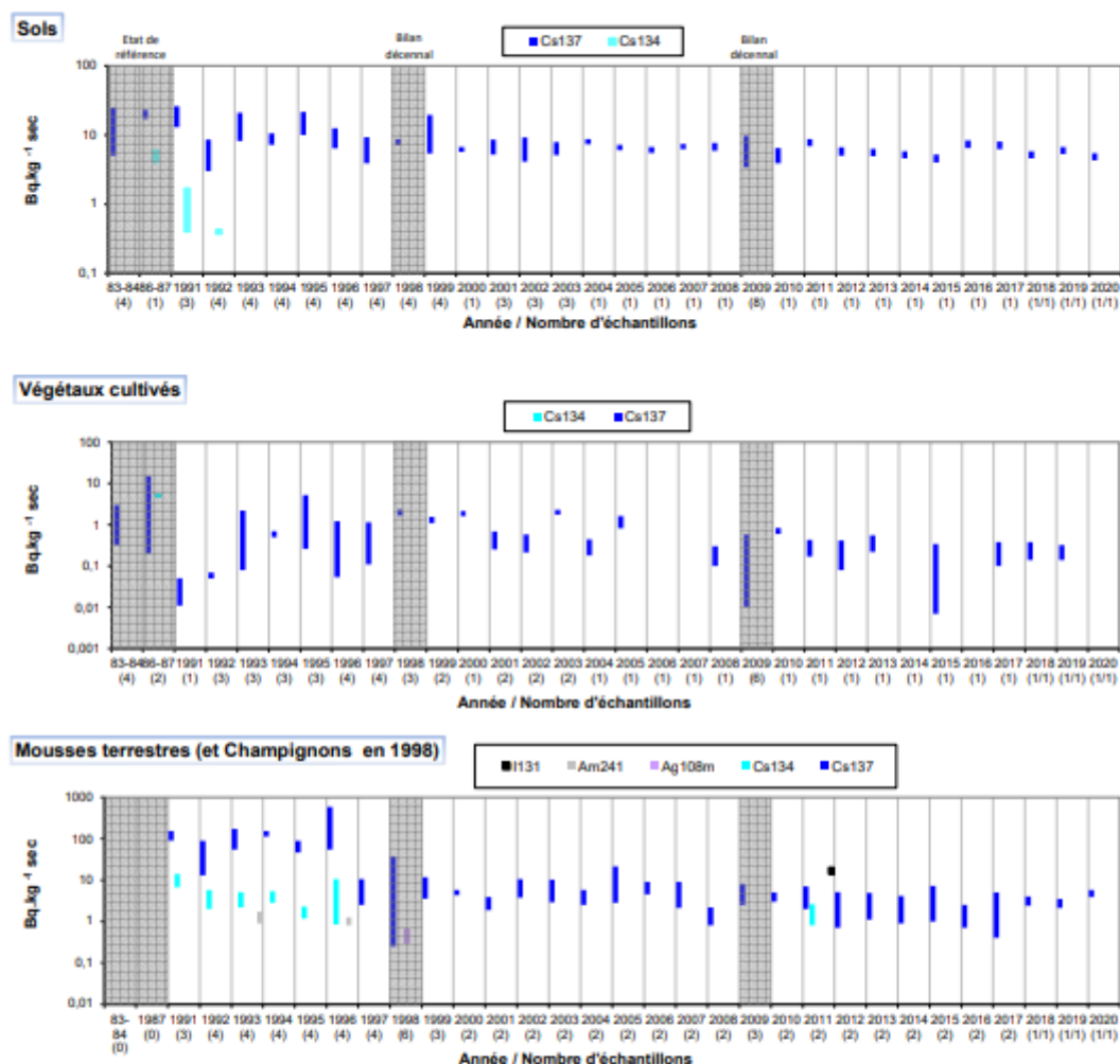
Figure 5-3. Gammes de variation (*) des activités des principaux radionucléides d'origine artificielle détectés par spectrométrie \gamma dans les échantillons prélevés dans le milieu terrestre de l'environnement du C.N.P.E. de Belleville-sur-Loire lors des études menées depuis l'état de référence de 1983/1984 au suivi radioécologique de 2020. (*) valeur minimale minorée de son incertitude à valeur maximale majorée de son incertitude
