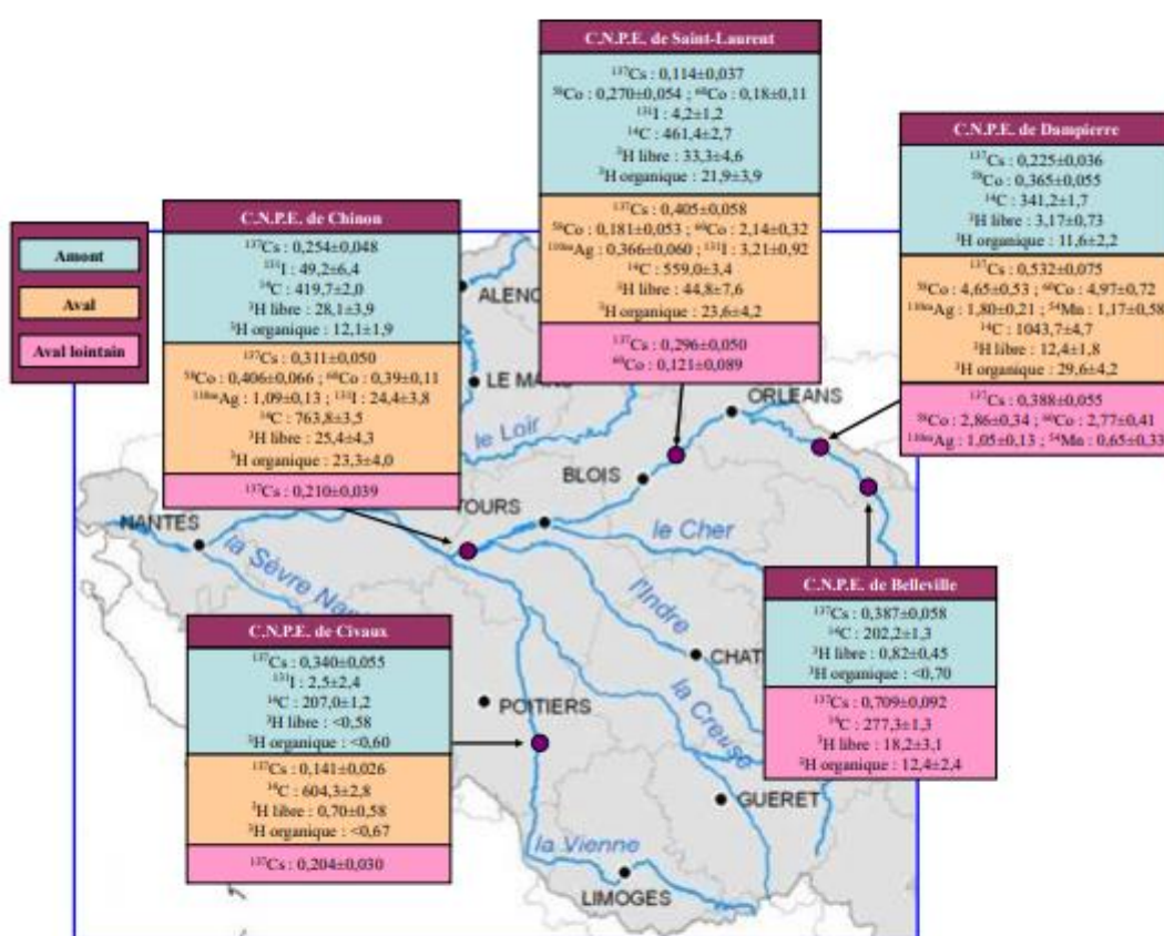
Figure 10-4. Synthèse des activités des radionucléides artificiels, du ^{14}\text{C} et du ^3\text{H} détectés dans les phanérogames et les mousses aquatiques prélevés en 2020 dans l'environnement des C.N.P.E. du bassin de la Loire.
