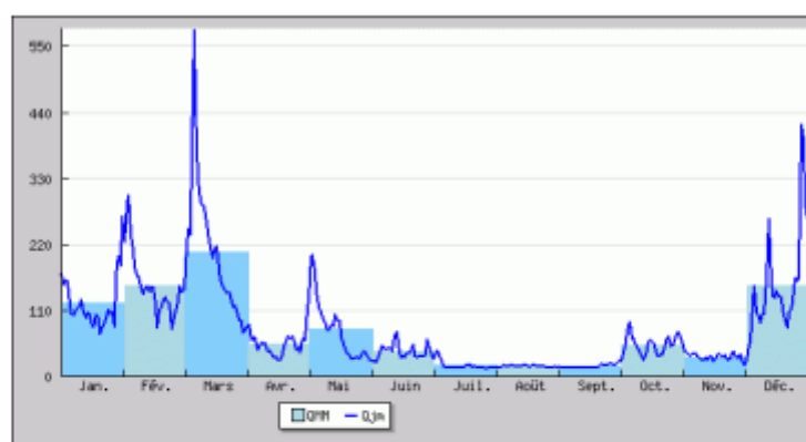
Figure 4-2. Hydrologie de la Vienne à la station de Lussac-les-Châteaux pour l'année 2020 (Qjm : débit moyen journalier en \text{m}^3.\text{s}^{-1} ; QMM : débit moyen mensuel en \text{m}^3.\text{s}^{-1} )
