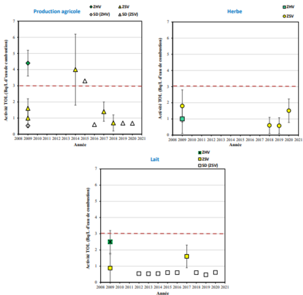
Figure 5-5. Activités en tritium organiquement lié dans les échantillons prélevés dans l'environnement terrestre du C.N.P.E. de Belleville-sur-Loire de 2009 à 2020. La ligne en pointillés représente la limite du bruit de fond ambiant hors influence industrielle ( <3 \text{ Bq.L}^{-1} ) [3,5].
