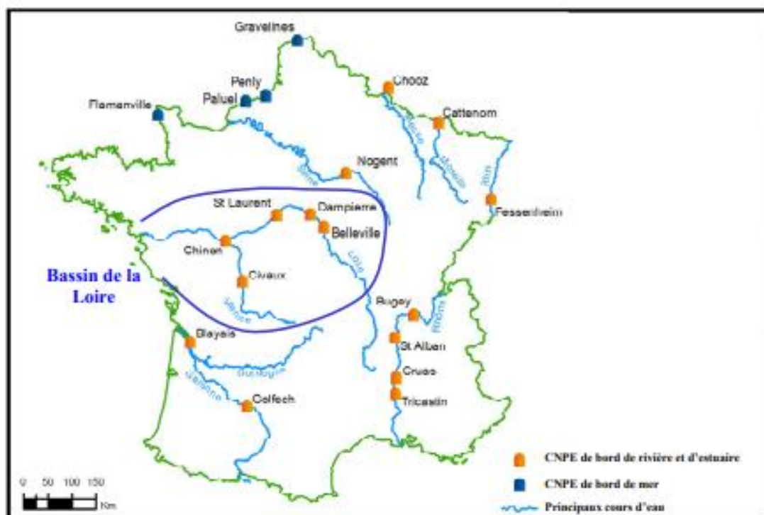
Répartition des C.N.P.E. français. – Identification des C.N.P.E. du bassin de la Loire.
