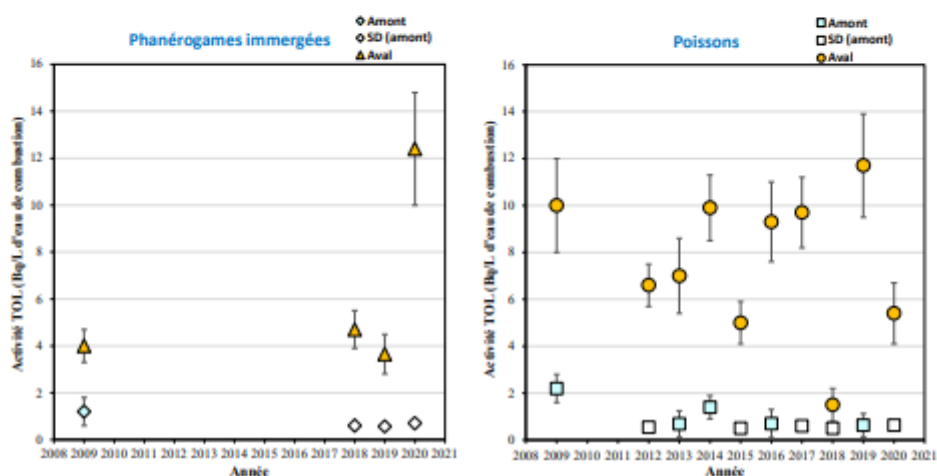
Figure 5-12. Activités en tritium organiquement lié dans les échantillons prélevés dans l'environnement aquatique du C.N.P.E. de Belleville-sur-Loire de 2009 à 2020.
