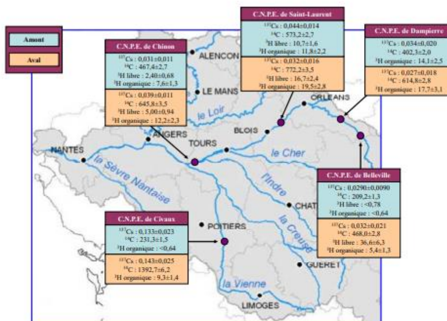
Figure 10-5. Synthèse des activités des radionucléides artificiels, du ^{14}\text{C} et du ^3\text{H} détectés dans les poissons prélevés en 2020 dans l'environnement des C.N.P.E. du bassin de la Loire.
