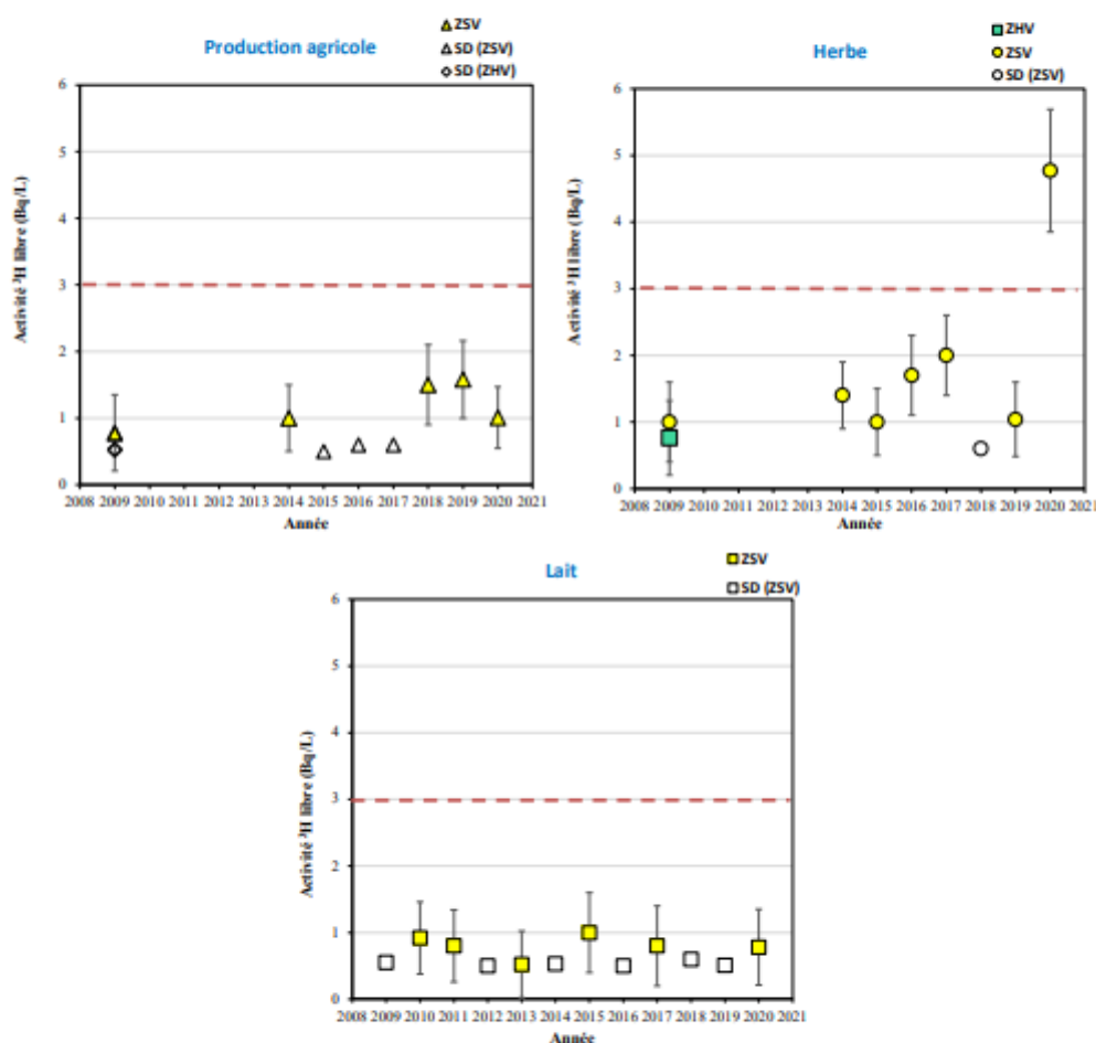
Figure 5-4. Activités en tritium libre dans les échantillons prélevés dans l'environnement terrestre du C.N.P.E. de Belleville-sur-Loire de 2009 à 2020.
