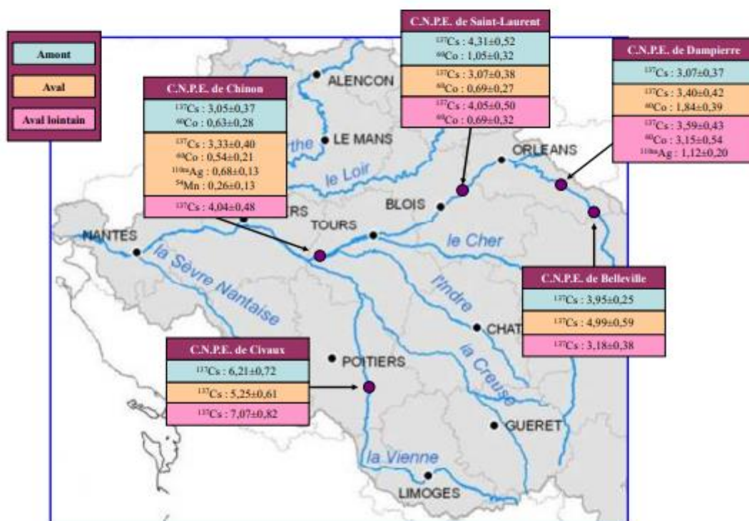
Figure 10-3. Synthèse des activités des radionucléides artificiels détectés dans les sédiments prélevés en 2020 dans l'environnement des C.N.P.E. du bassin de la Loire ( \text{Bq.kg}^{-1} sec).
