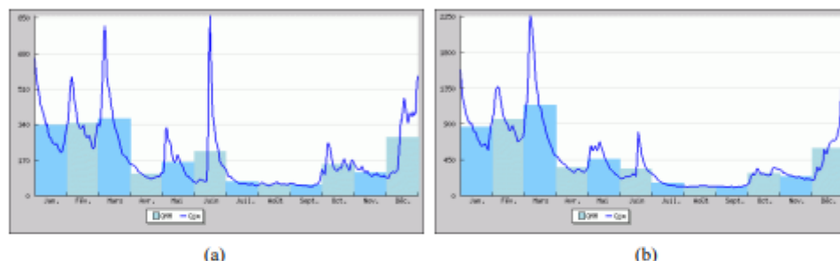
Figure 4-1. Hydrologie de la Loire à la station de Saint-Satur (a) et à la station de Saumur (b) pour l'année 2020 (Qjm : débit moyen journalier en \text{m}^3.\text{s}^{-1} ; QMM : débit moyen mensuel en \text{m}^3.\text{s}^{-1} )
