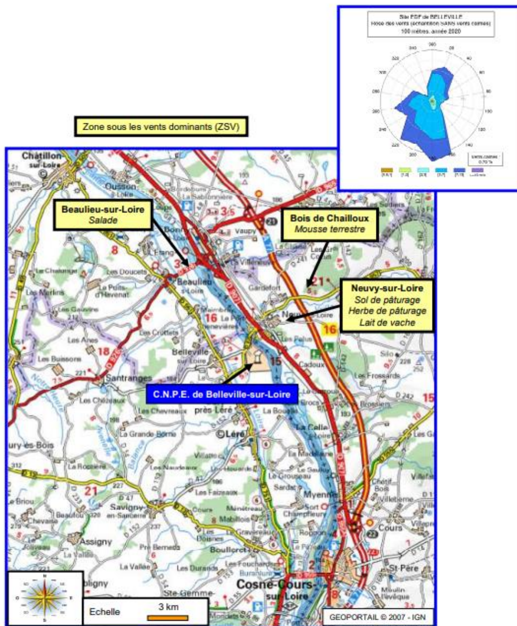
Figure 5-2. Stations et natures des prélèvements du milieu terrestre pour le suivi radioécologique 2020 du C.N.P.E. de Belleville-sur-Loire.
