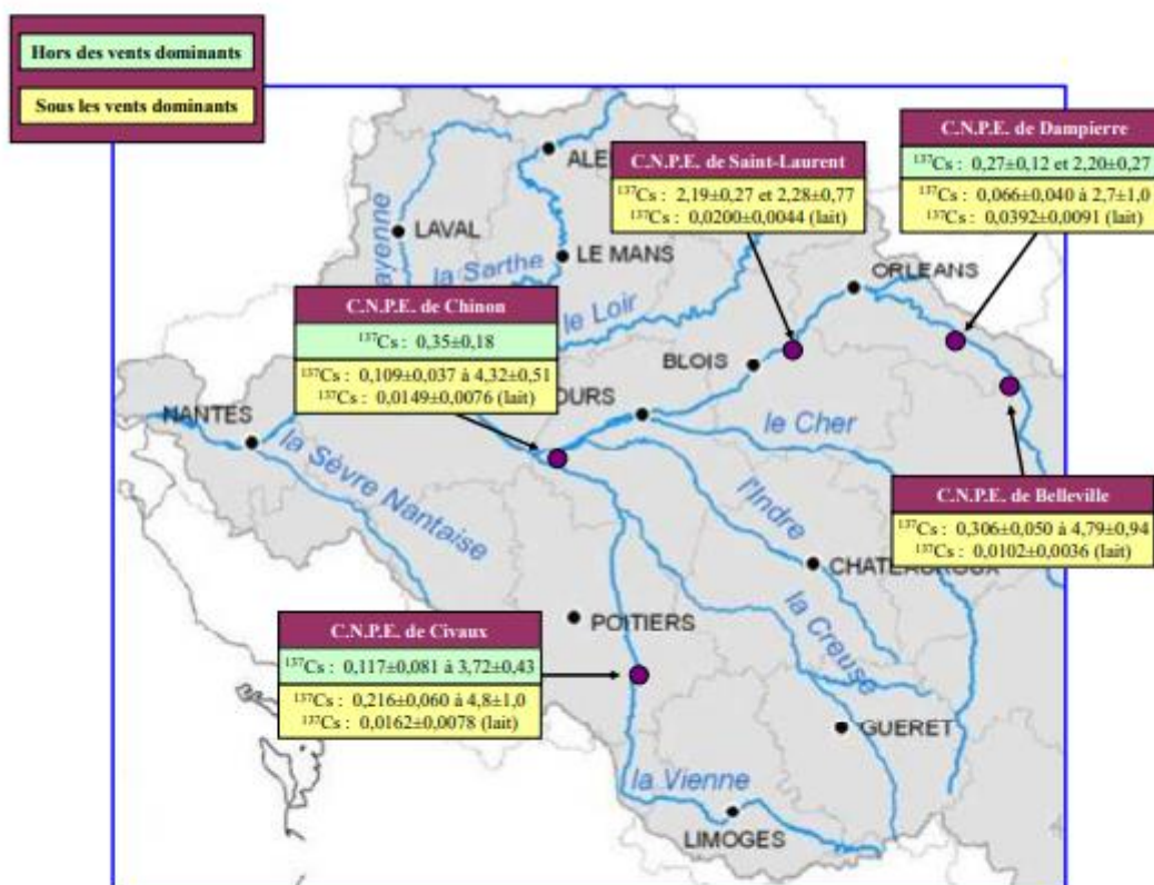
Figure 10-1. Synthèse des activités des radionucléides artificiels émetteurs gamma détectés dans les échantillons prélevés en 2020 dans l'environnement terrestre des C.N.P.E. du bassin de la Loire.
