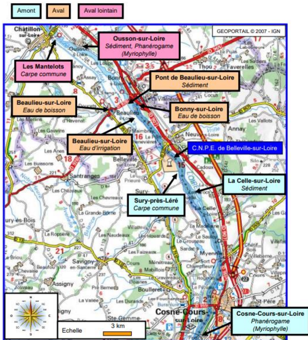
Figure 5-7. Stations et natures des prélèvements du milieu aquatique pour le suivi radioécologique 2020 du C.N.P.E. de Belleville-sur-Loire.
