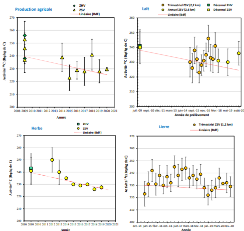
Figure 5-6. Activités spécifiques en ^{14}\text{C} mesurées dans les échantillons prélevés dans l'environnement terrestre du C.N.P.E. de Belleville-sur-Loire de 2009 à 2020.
