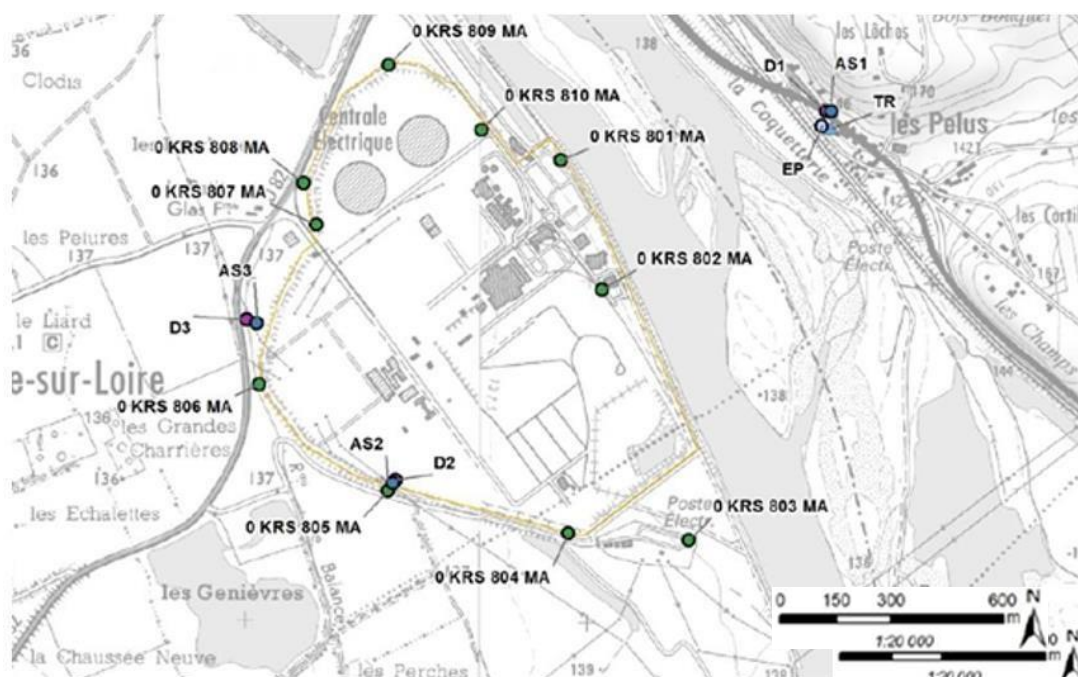
Figure 5 : Localisation des stations KRS (réseaux clôture et 1km)
