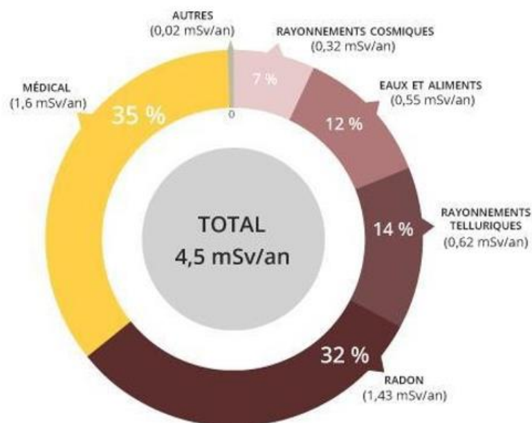
Figure 7 : Part relative des différentes sources d'expositions de la population française aux rayonnements ionisants (Source : Bilan IRSN 2015)
