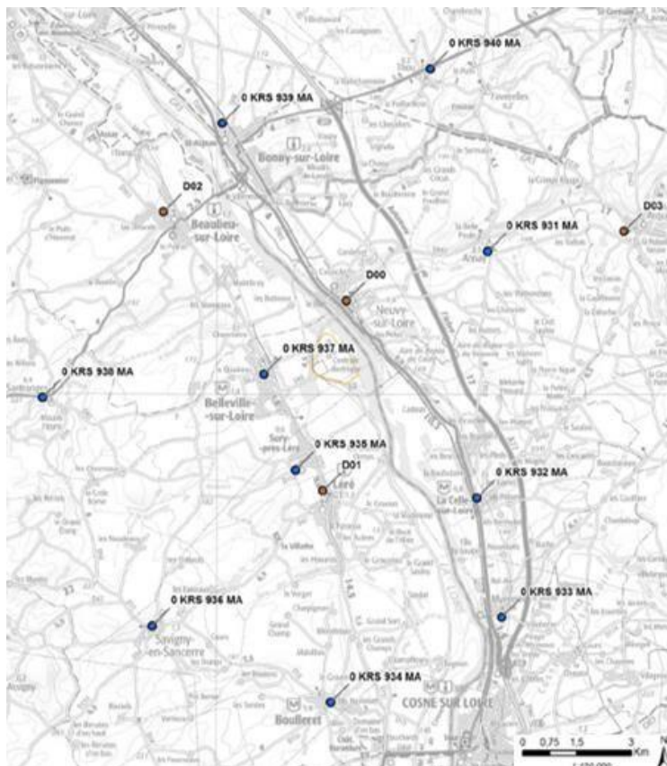
Figure 4 : Localisation des stations KRS (réseaux 5 et 10 km)
