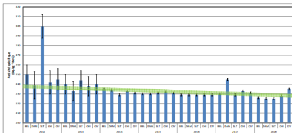
Figure 10-2. Activités spécifiques en ^{14}\text{C} mesurées dans les herbes de pâturage prélevées dans l'environnement terrestre des C.N.P.E. du bassin de la Loire de 2012 à 2018. Le bandeau vert représente le bruit de fond ambiant hors influence industrielle ( 227 \text{ Bq.kg}^{-1} de C).
