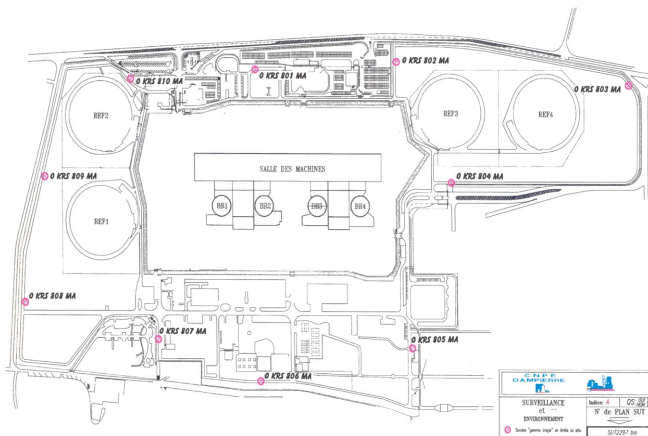
Réseau de balises radiamétriques « clôture »
