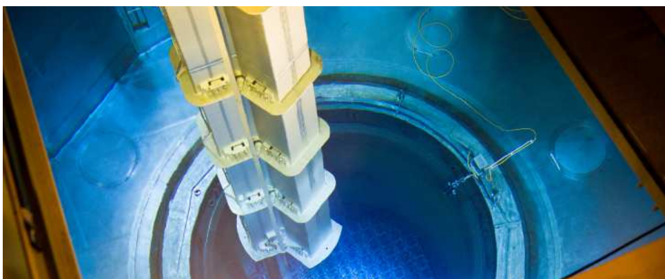
Photo prise par David Queyrel, salarié à la centrale de Cattenom, pendant l'opération de déchargement du combustible sur l'unité de production n°3.
